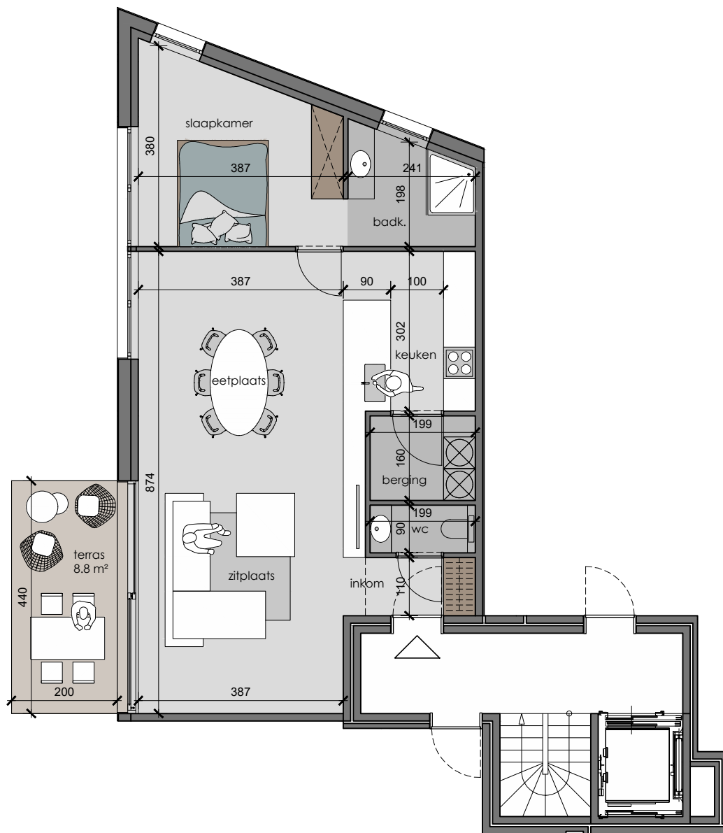
Verdieping 1 - appartement 1.6 netto oppervlakte 70.7 m 2 - bruto oppervlakte 79.8 m 2 opp. terras 8.8 m 2
